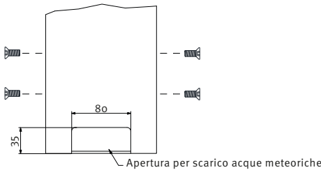
prospetto
