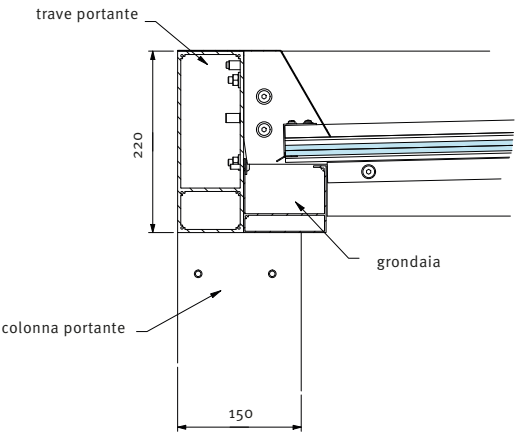
dettaglio
